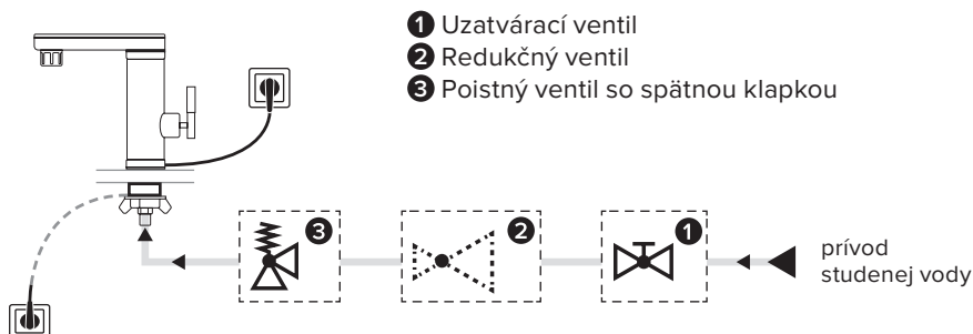
obr. 3: odporúčané zapojenie priamoohrevnej batérie na plný tlak vody do vodovodného systému.
